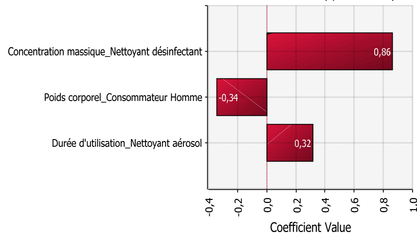
DI totale_Nettoyant aérosol_Homme adulte Correlation Coefficients (Spearman Rank)
