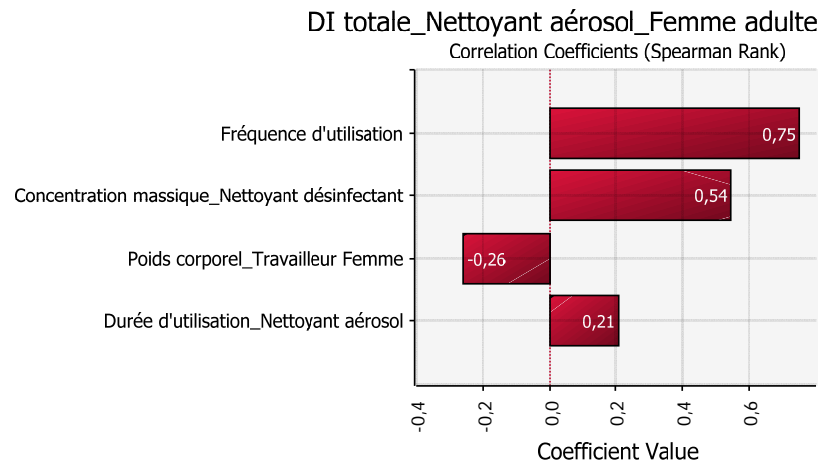
Analyse de sensibilité – tornado graph
