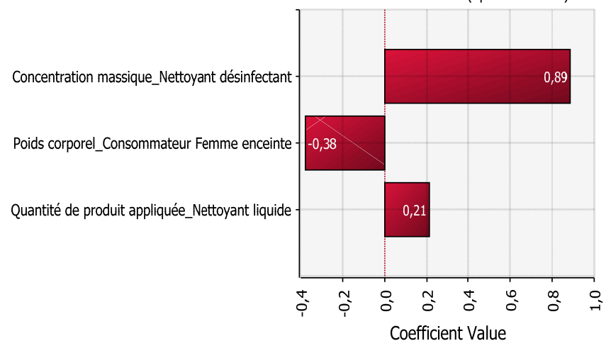
DI totale_Nettoyant liquide_Femme enceinte Correlation Coefficients (Spearman Rank)
